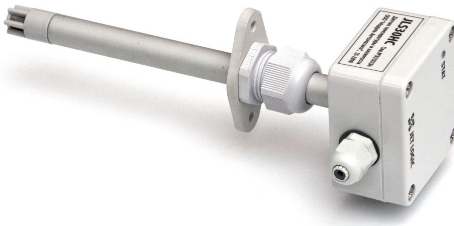
Рис. 1 - Датчик JLS30HC
