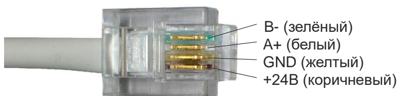
Рис. 10 - Расположение сигналов на RJ-14
