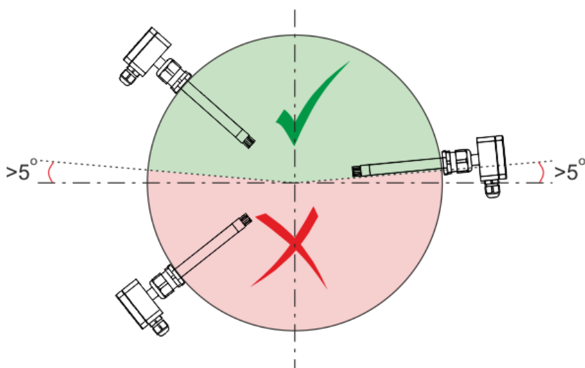
Рис. 8 - Монтаж датчика на круглый воздуховод
