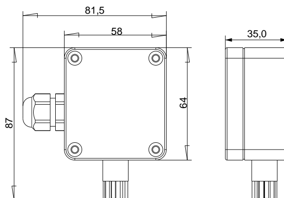
Рис. 6 - Габаритные размеры датчика JLS30HW
