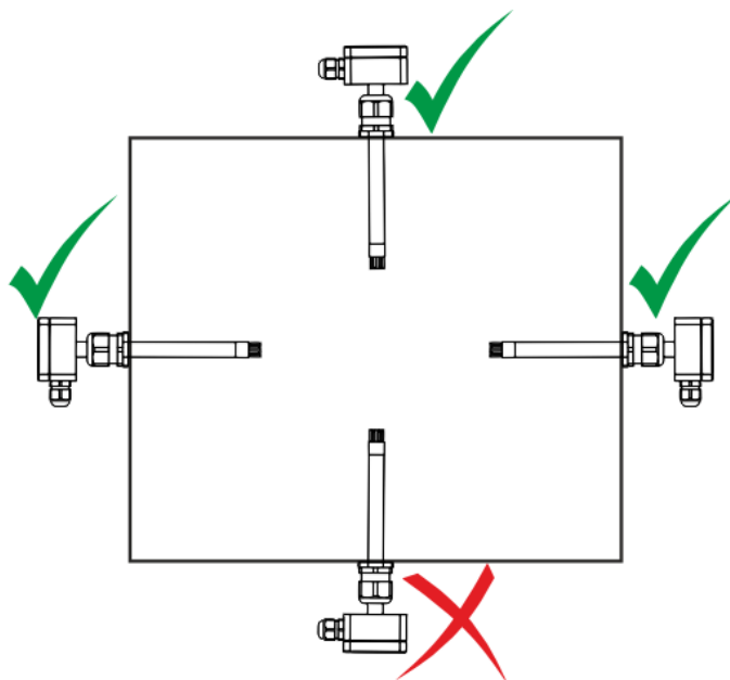
Рис. 7 - Монтаж датчика на прямоугольный воздуховод
