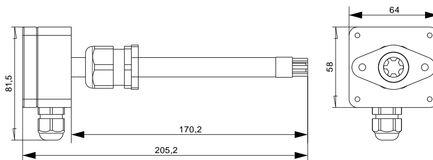
Рис. 5 - Габаритные размеры датчика JLS30HC
