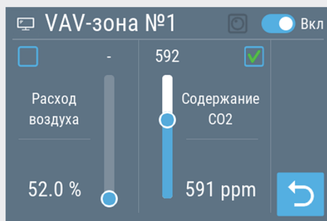
Новый пульт JLV135 с расширенными возможностями по управлению VAV-системами
